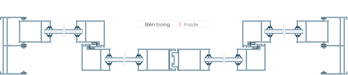
Mặt cắt ngang | Horizontal section
