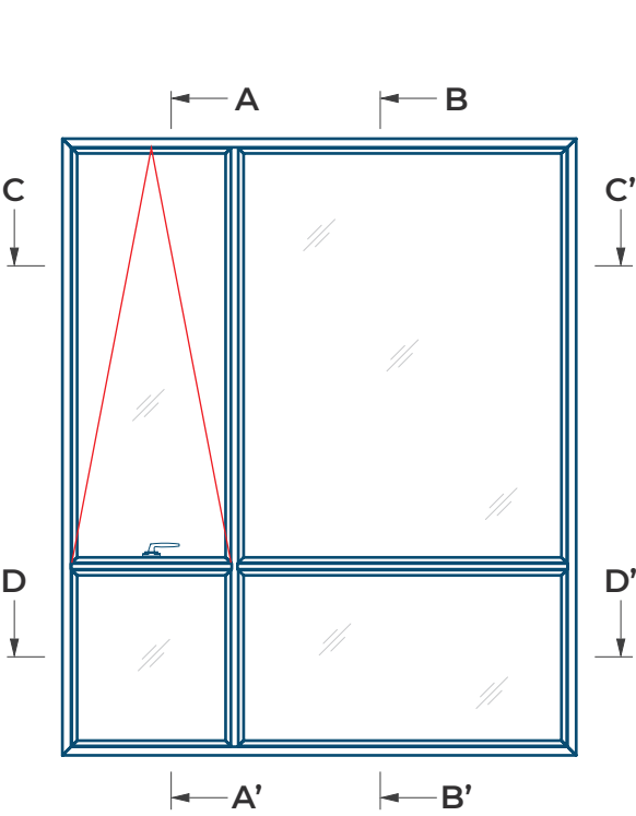
Chi tiết | Details
