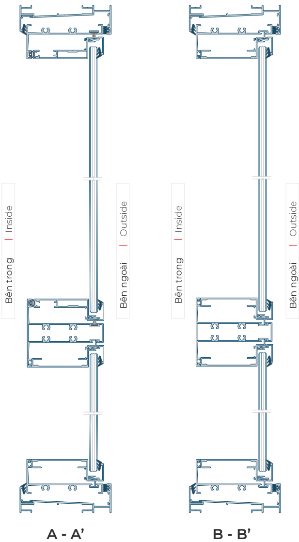
Mặt cắt dọc | Vertical section
