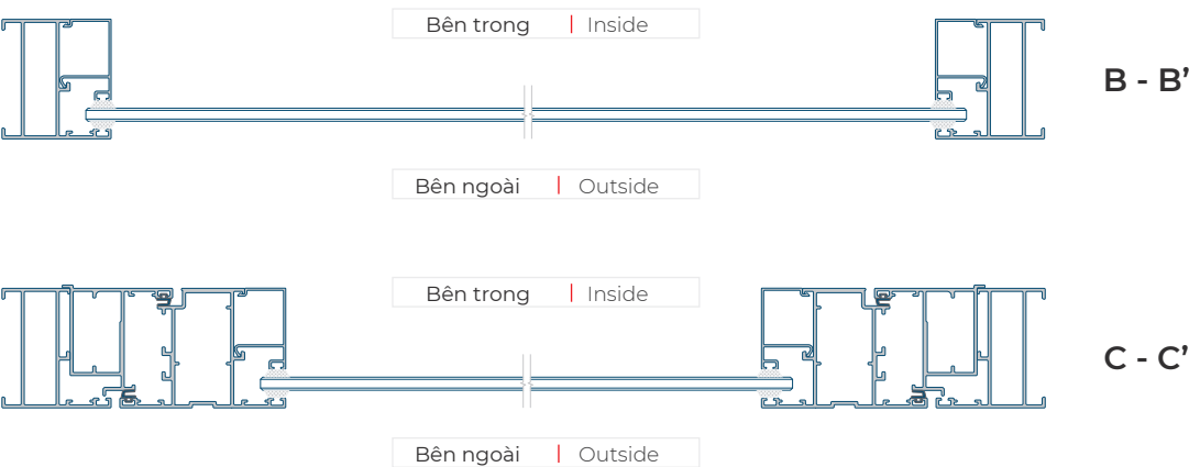
Mặt cắt ngang | Horizontal section
