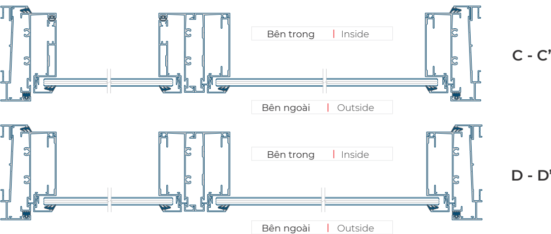
Mặt cắt ngang | Horizontal section
