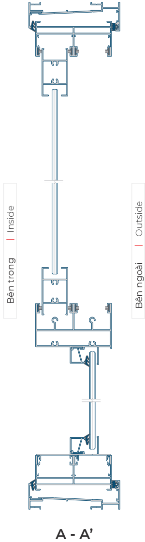
Mặt cắt dọc | Vertical section
